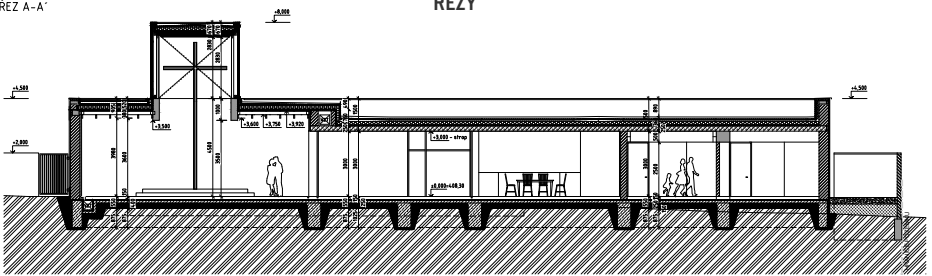
ŘEZ A-A'
